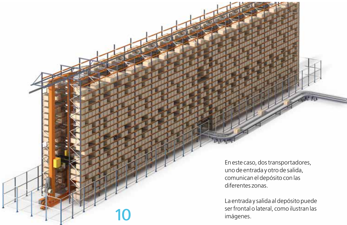
Depósito automático para cajas de cartón con entrada y salida lateral.
