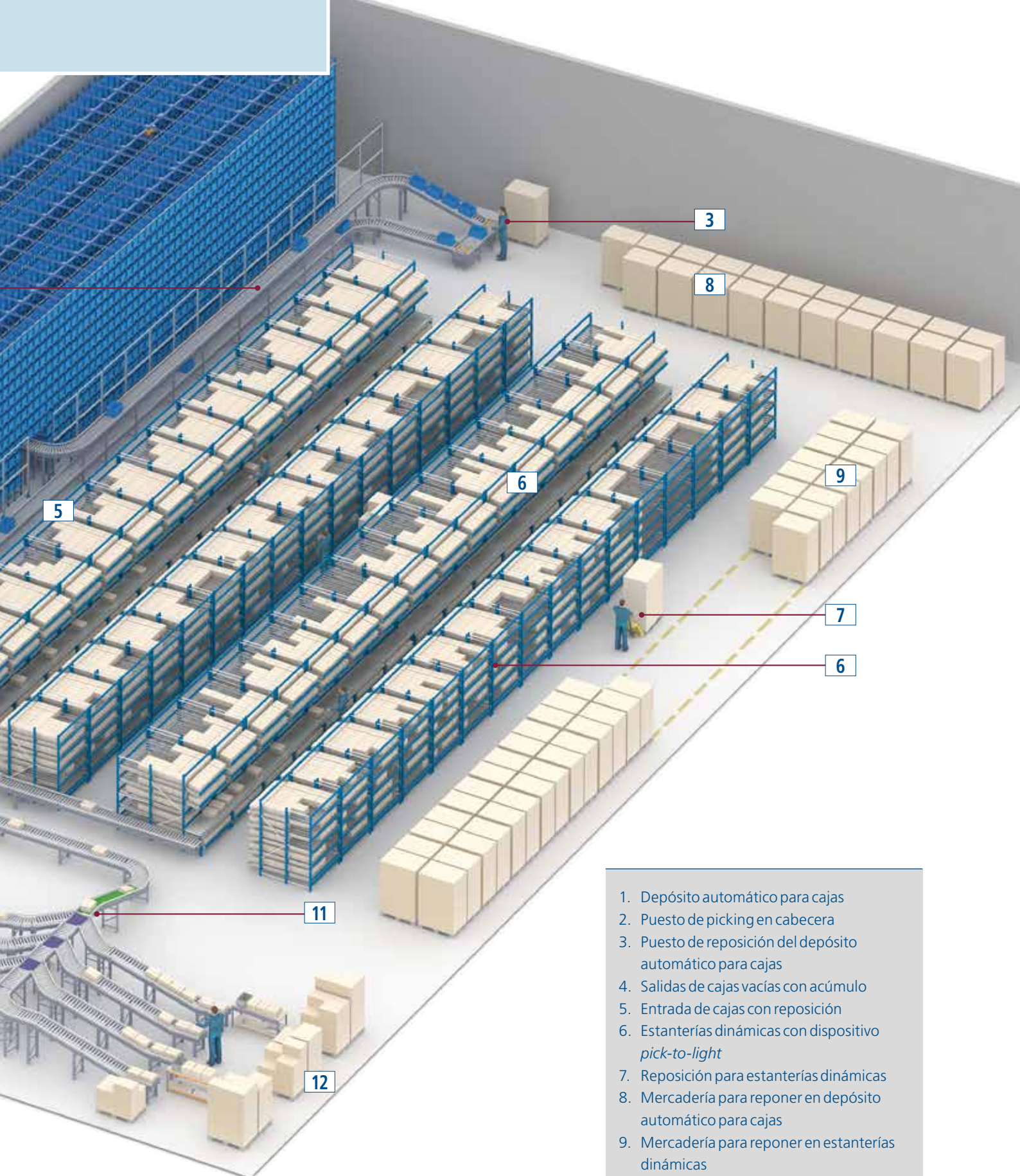
Depósito automático para cajas combinado con estanterías dinámicas y un clasificador de pedidos.
