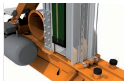
Detalle de la unión de la columna con el testero inferior.
